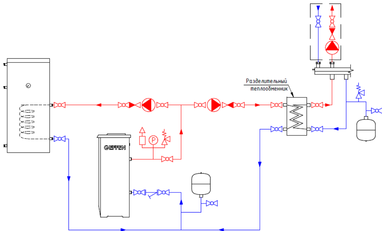
Схема подключения котла в существующую/реконструируемую систему отопления
